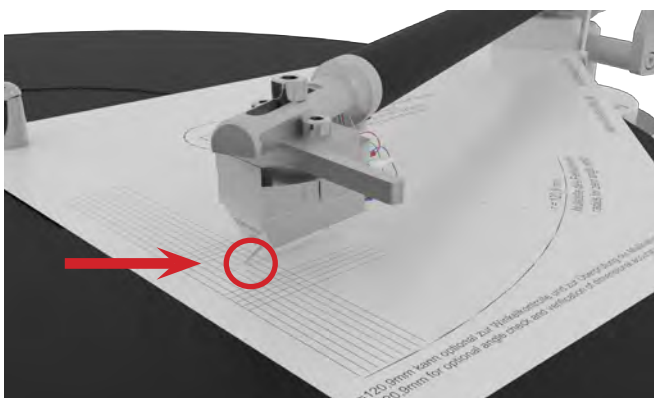
Abb. 12: Korrekte Position des Abtastdiamanten
