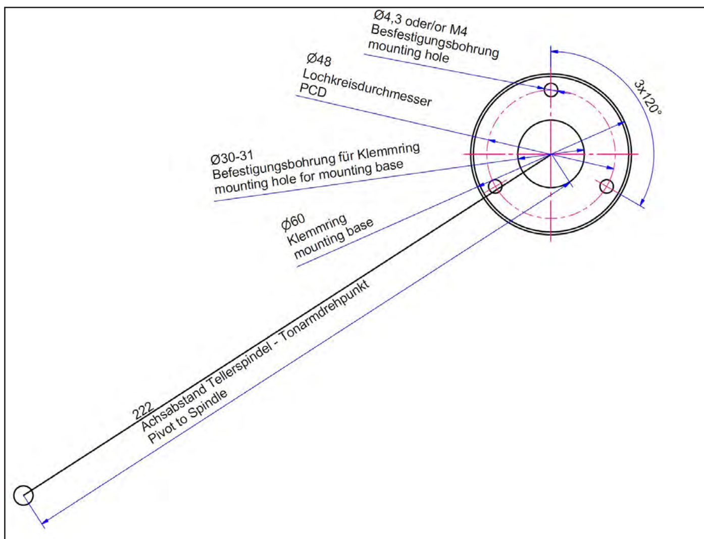
Abb. 3: Bohrschablone für die Montage des Klemmrings auf einem Laufwerk eines anderem Herstellers
